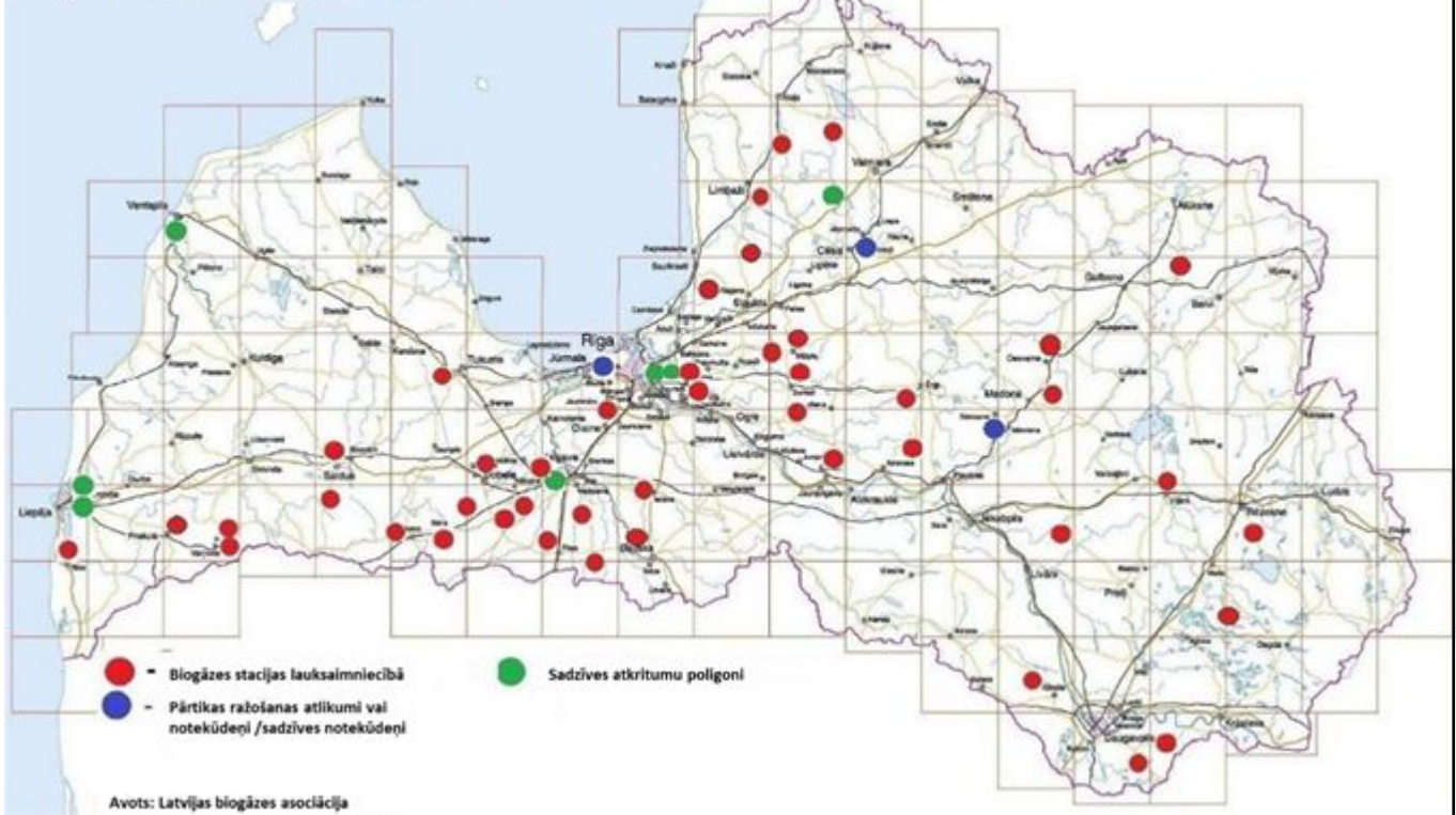
15.attēls. Biogāzes stacijas Latvijā 2014.gada 1.jūlijā. Avots: Latvijas Biogāzes asociācijas dati
